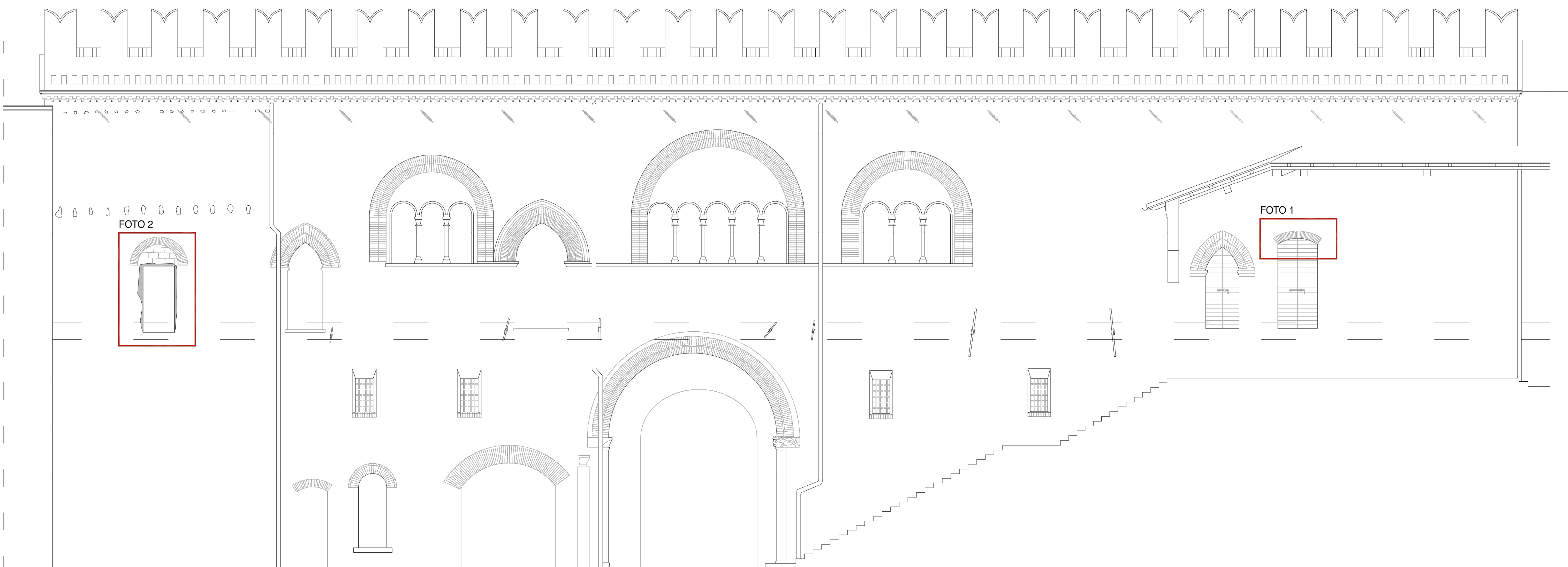
PROSPETTO FABBRICATO SU PIAZZA DEI MARTIRI
