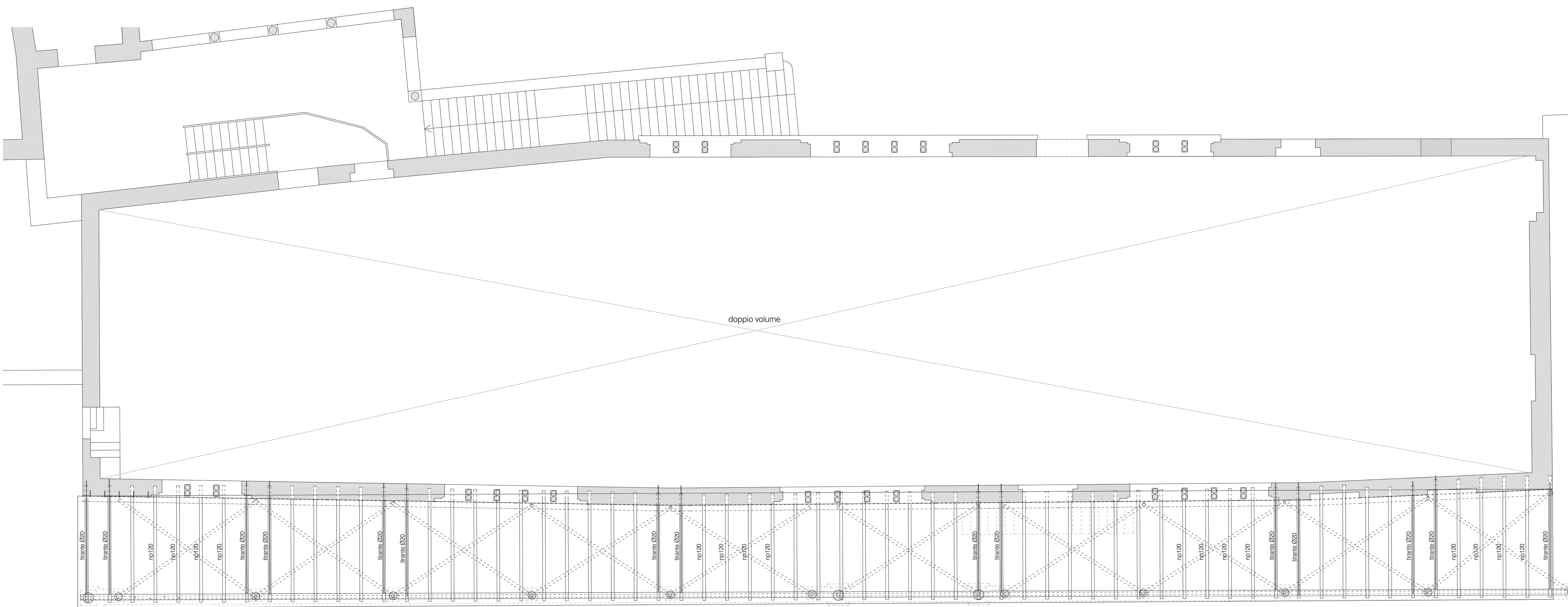
PIANTA PIANO SECONDO - SALONE DELL'ARENGO
