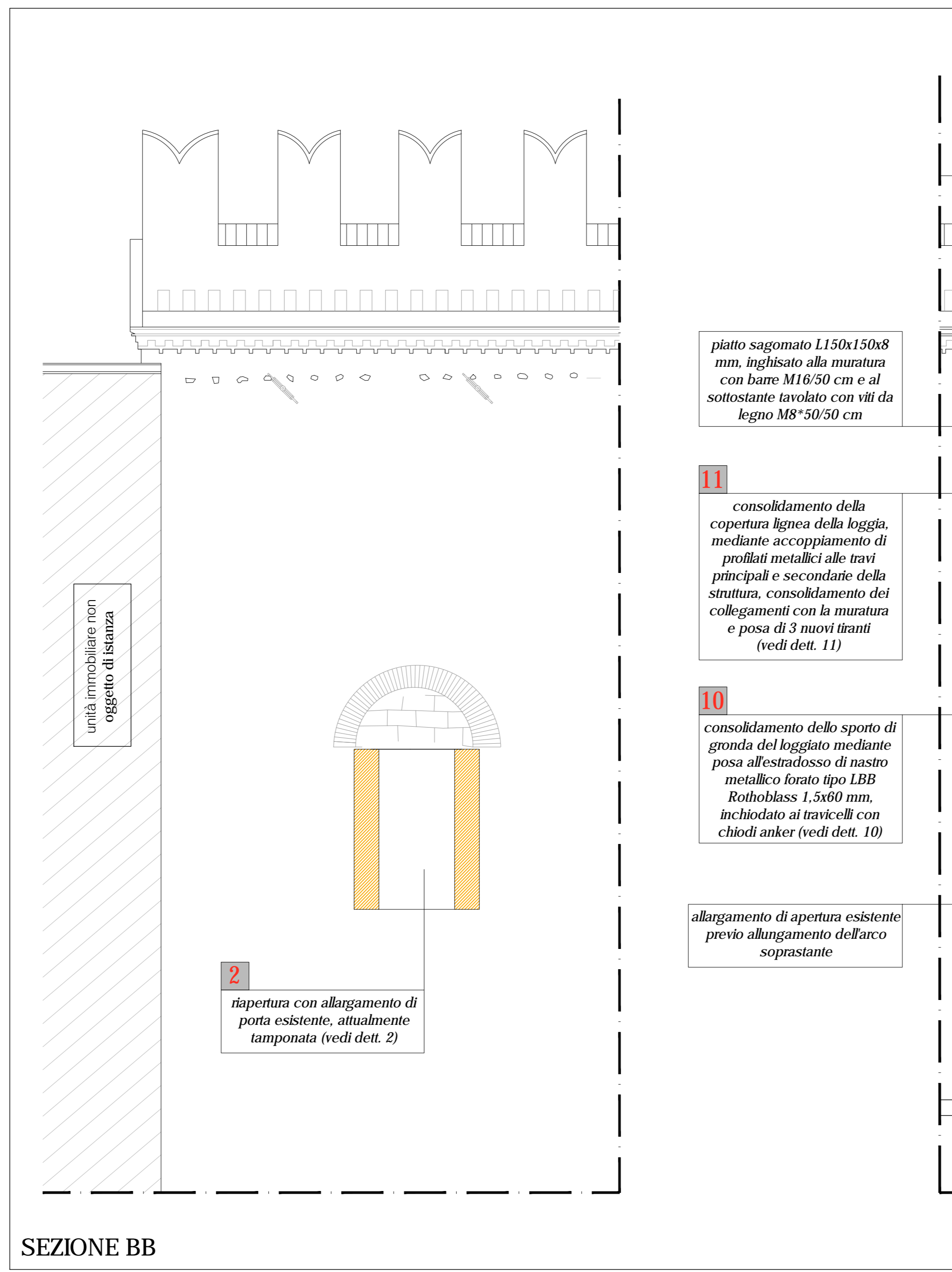
SEZIONE BB
