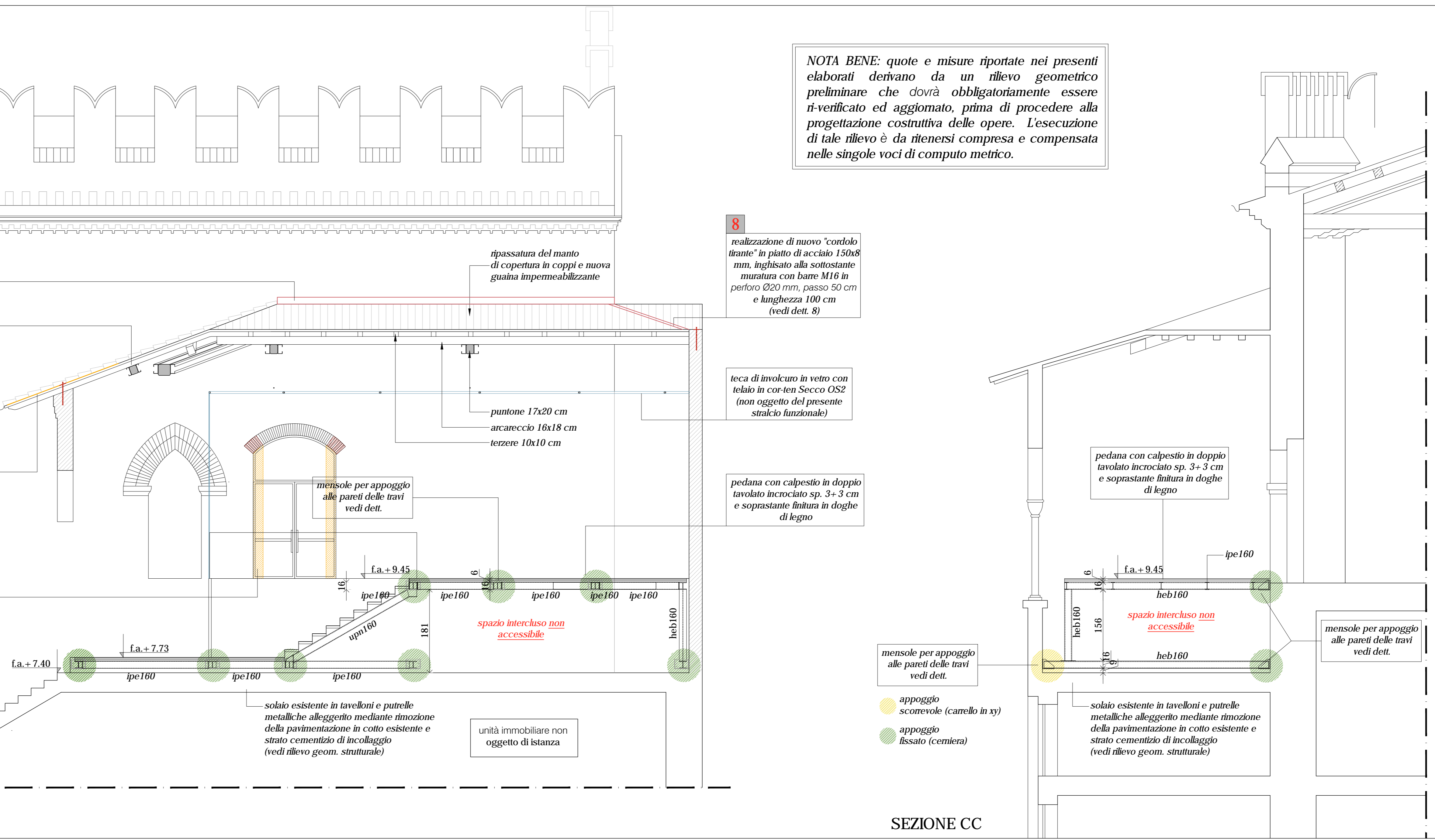
SEZIONE CC
