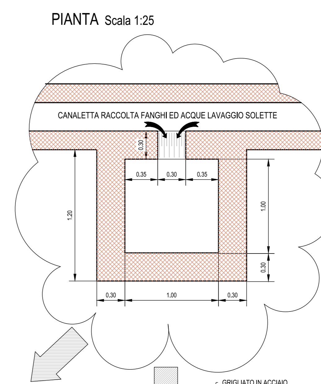
POZZETTO PER RACCOLTA E SOLLEVAMENTO ACQUE DI LAVAGGIO SOLETTE E CANALETTA
