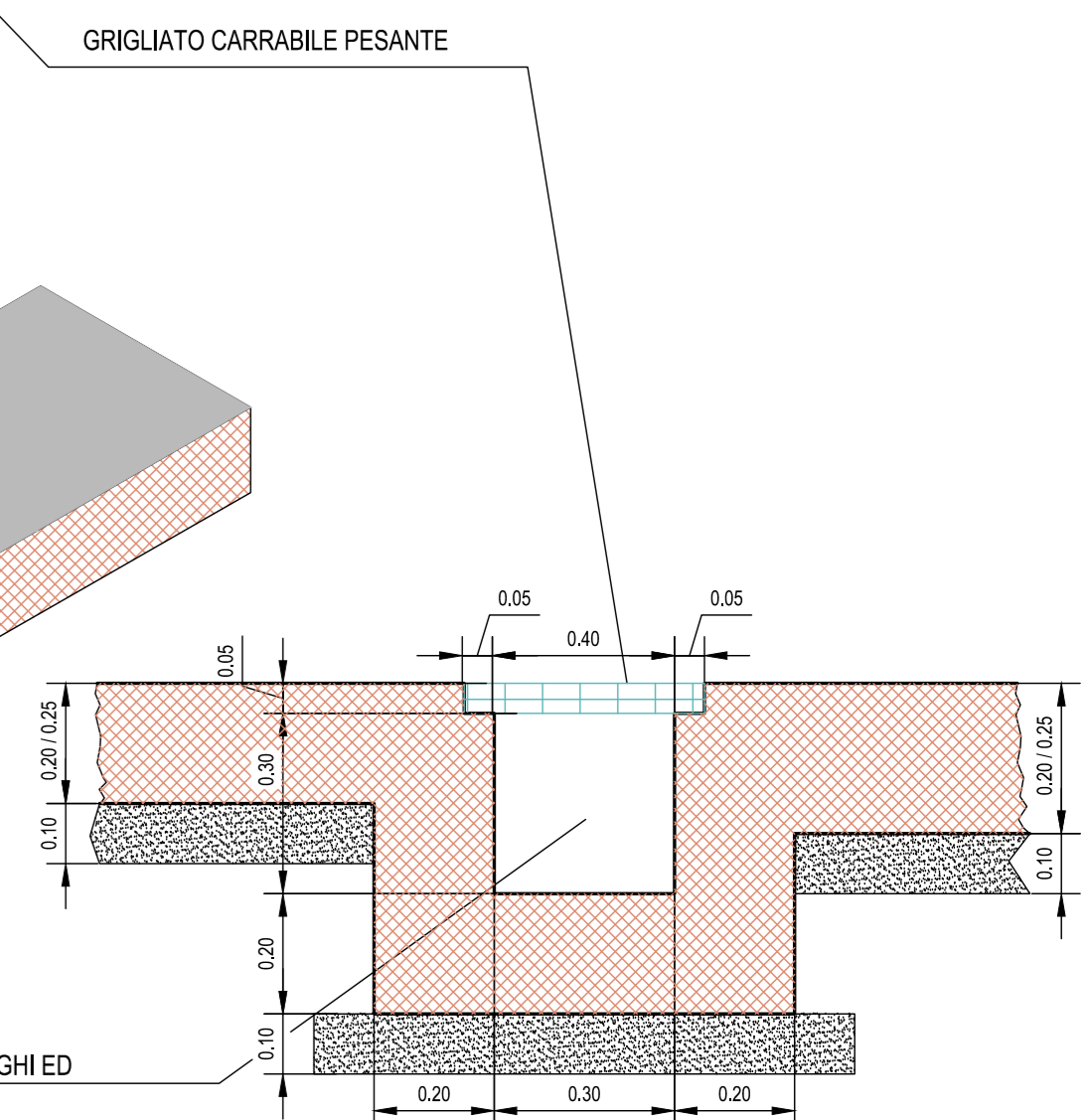
SEZIONE CANALETTA INTERNA Scala 1:12,5
