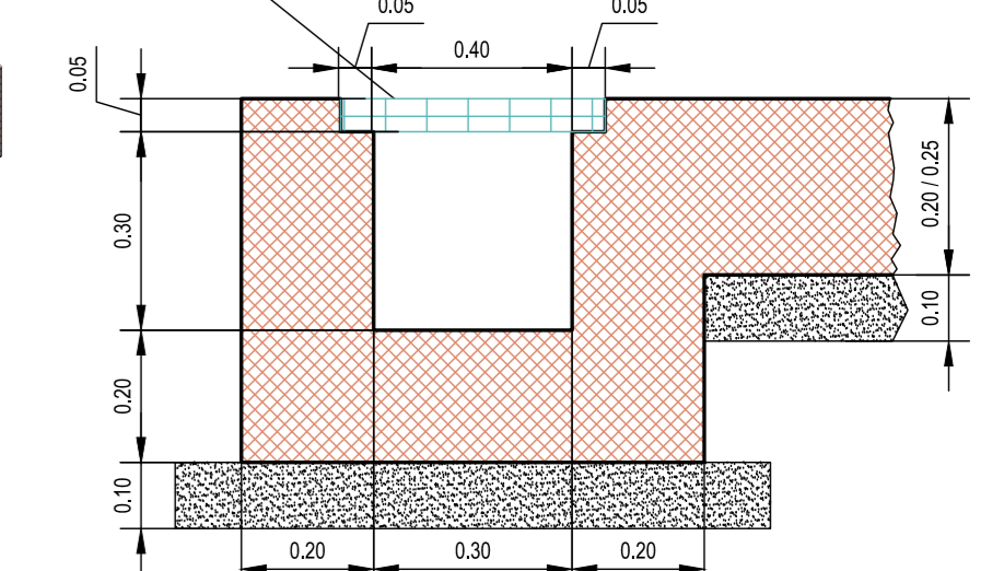
SEZIONE CANALETTA DI BORDO Scala 1:12,5
