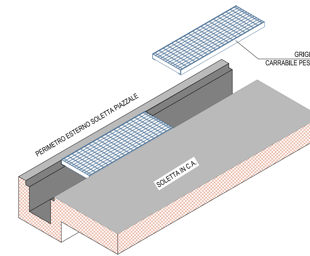
PARTICOLARE CANALETTA DI BORDO
