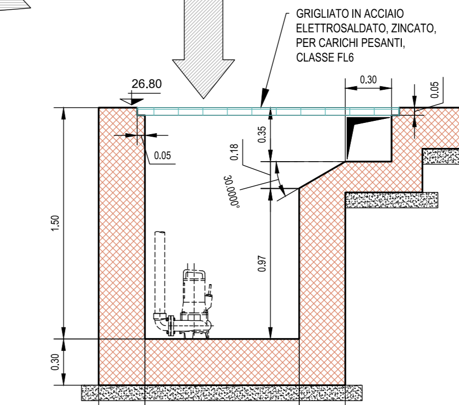
SEZIONE H - H Scala 1:25
