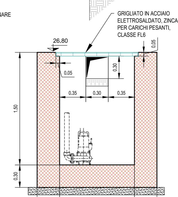
SEZIONE G - G Scala 1:25
