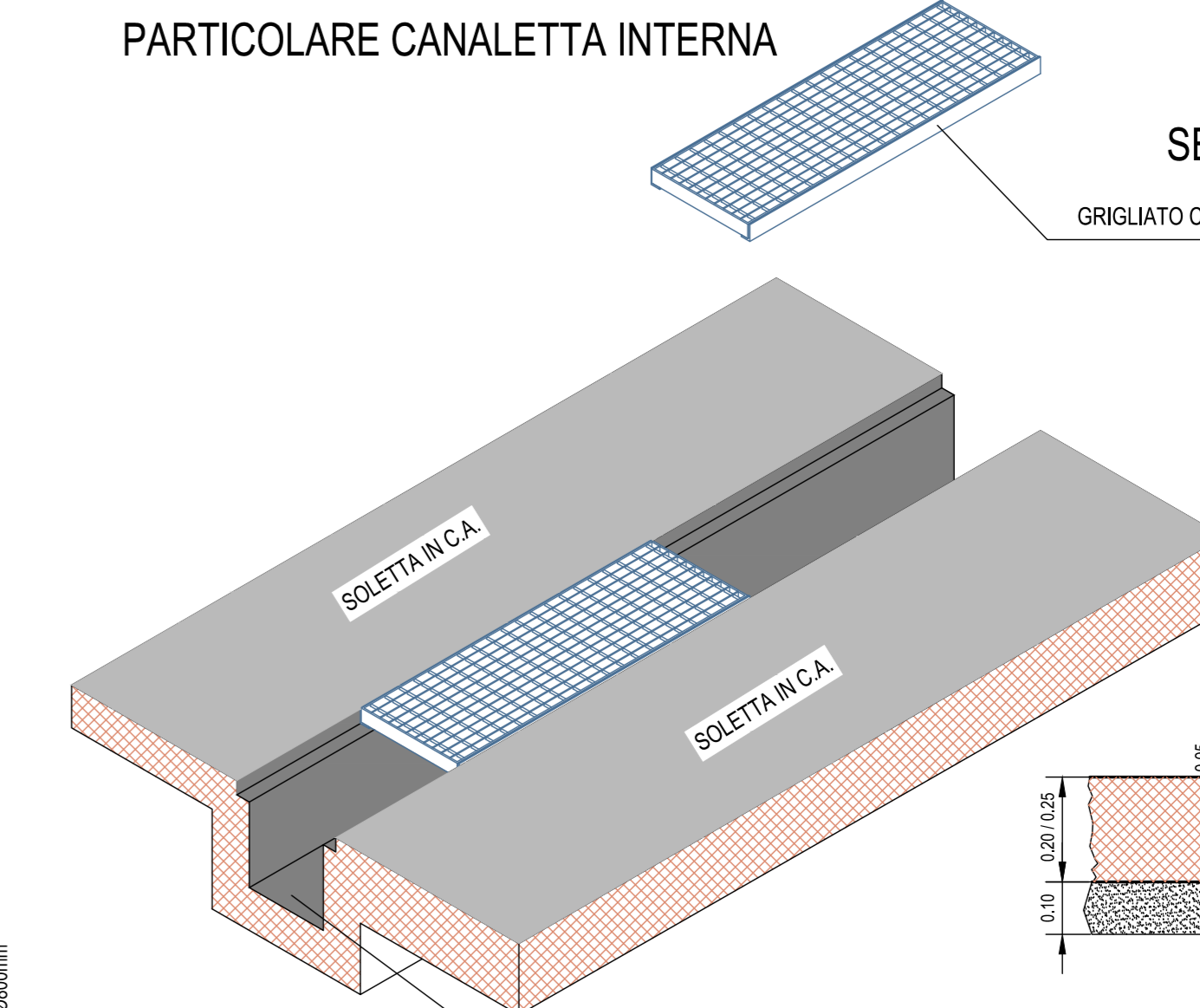
PARTICOLARE CANALETTA INTERNA
