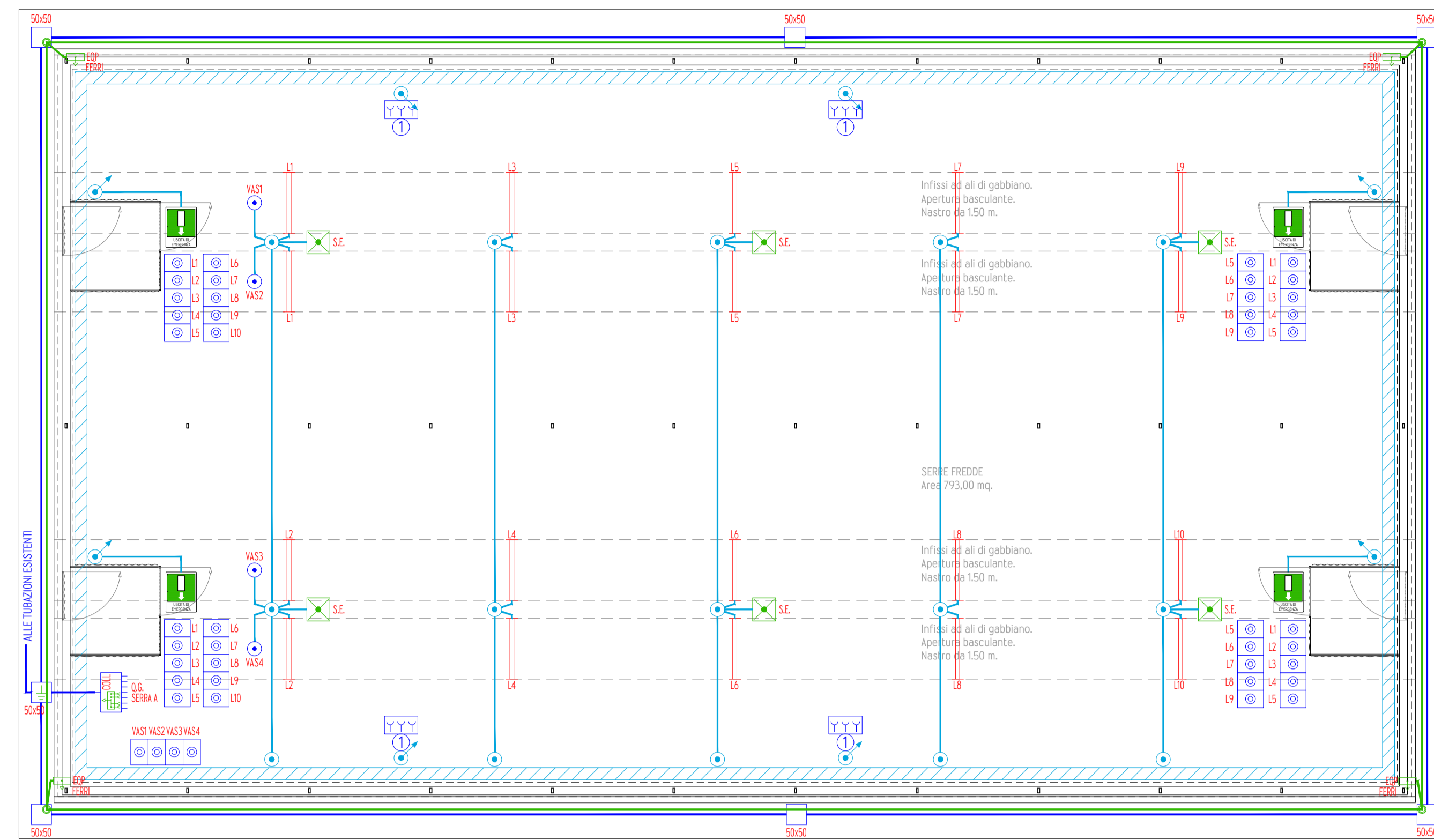
Particolare serra A - scala 1:100
