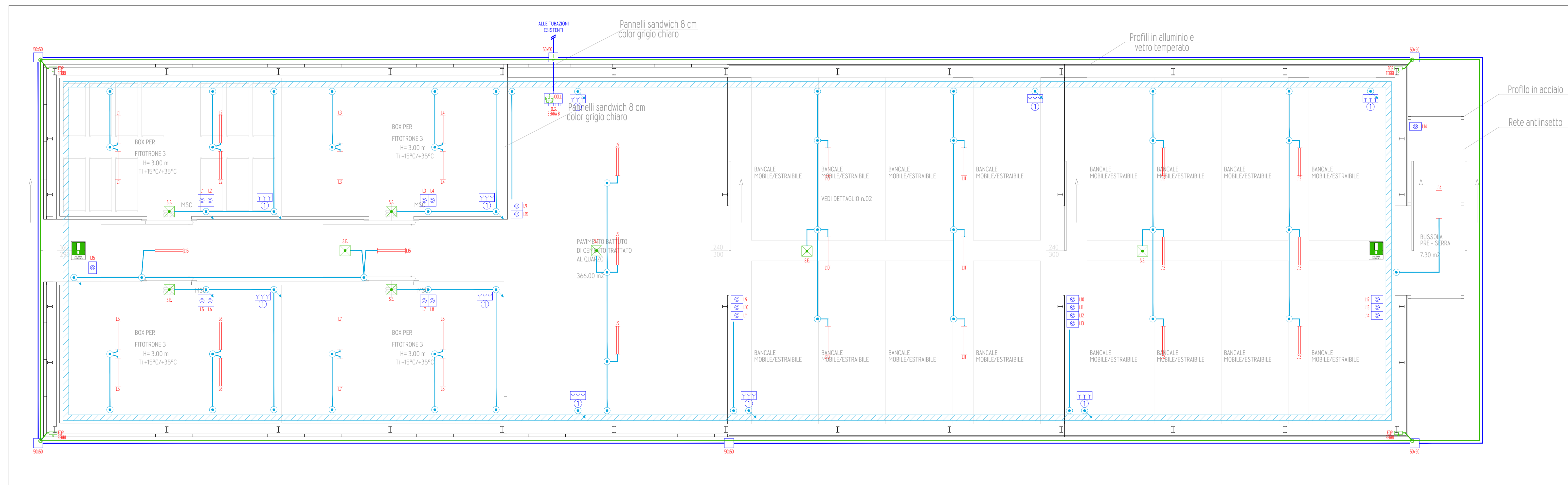
Particolare serra B - scala 1:50
