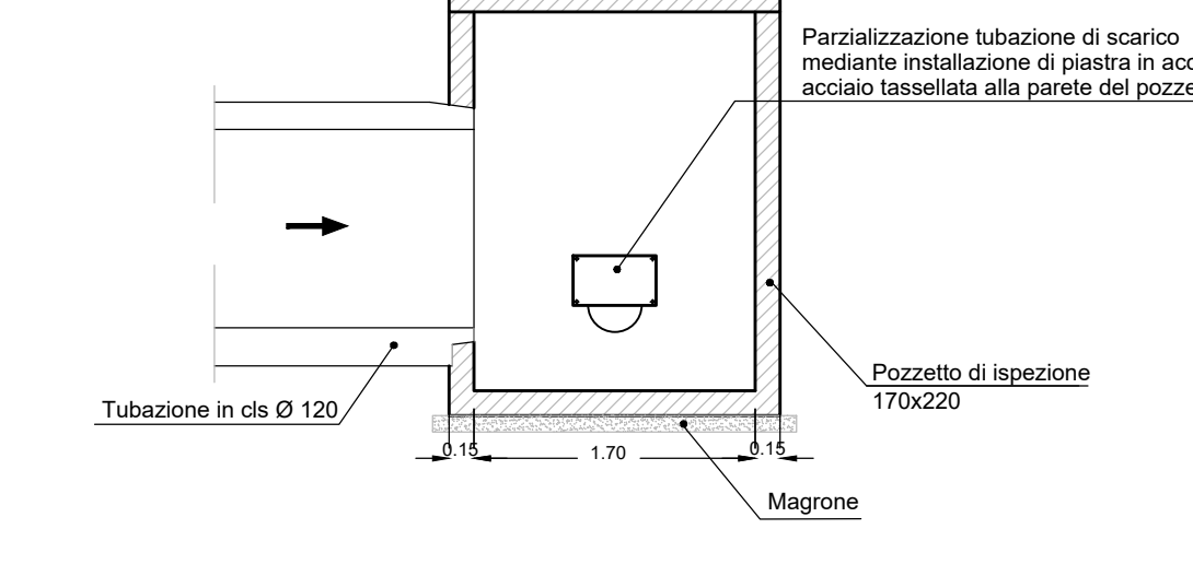
PARTICOLARE SEZIONE C-C Scala 1:50
