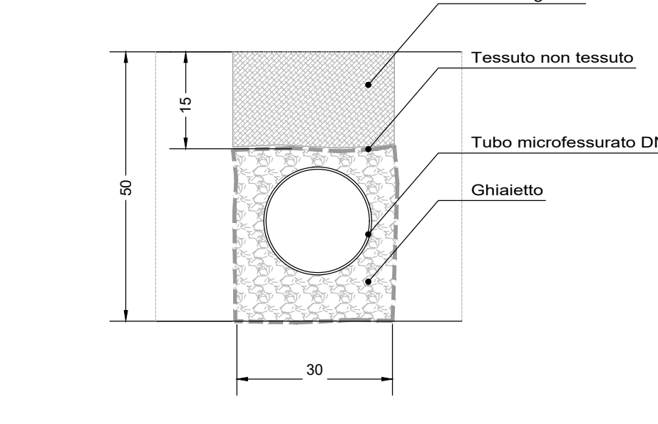
PARTICOLARE DRENAGGIO FONDO SEZIONE Z-Z Scala 1:10
