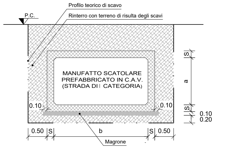
SEZIONE TRASVERSALE TIPO ELEMENTI SCATOLARI PREFABBRICATI IN C.A.V. CON GIUNTO A BICCHIERE ED ANELLO DI TENUTA IN GOMMA SINTETICA Scala 1:50
