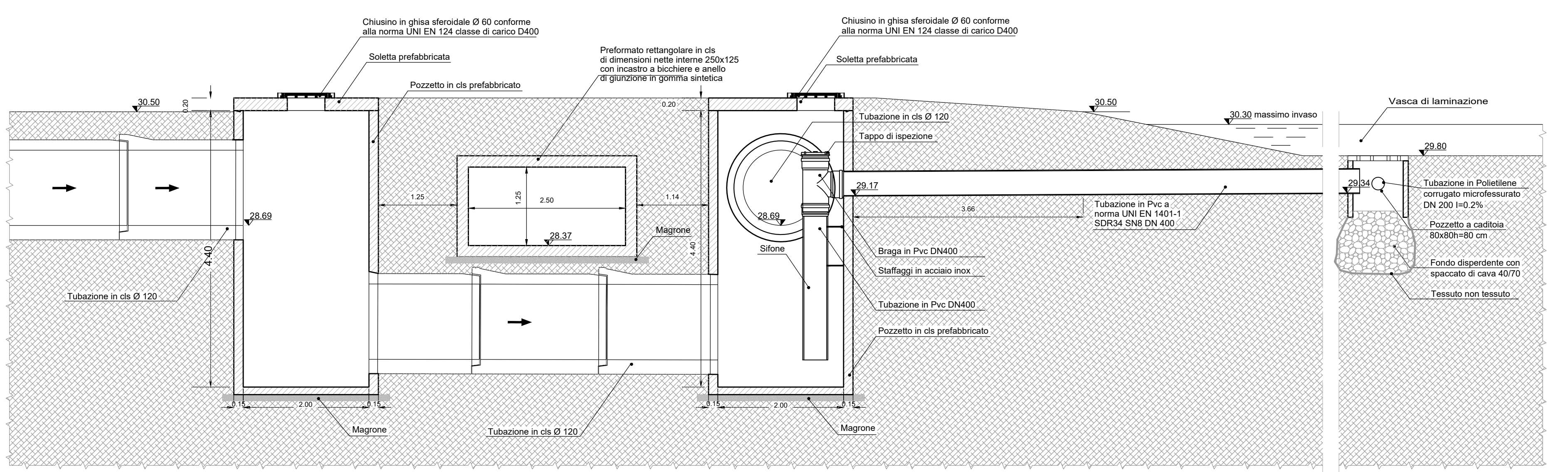
PARTICOLARE "A" Scala 1:50
