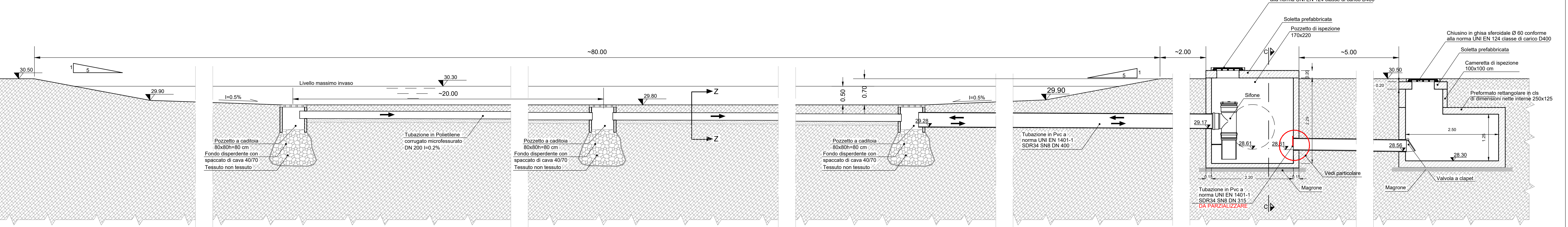
PARTICOLARE SEZIONE A-A VASCA DI LAMINAZIONE- BACINO 2 Scala 1:50
