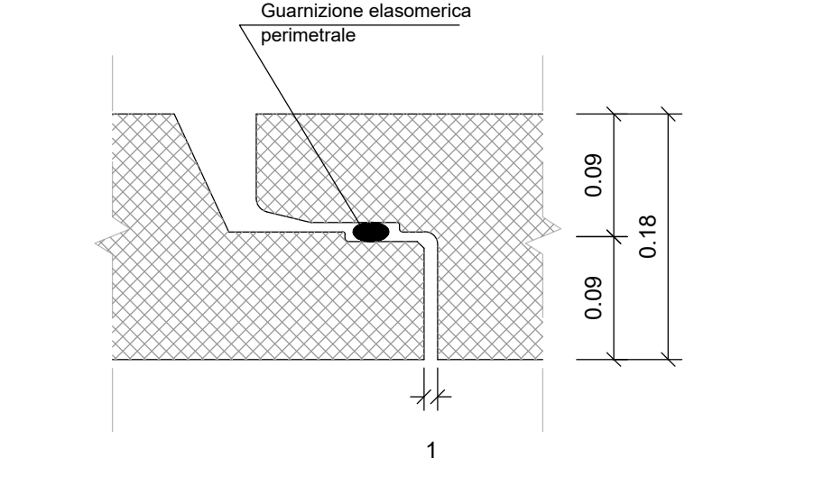
PARTICOLARE GIUNZIONI ELEMENTI SCATOLARI Scala 1:10
